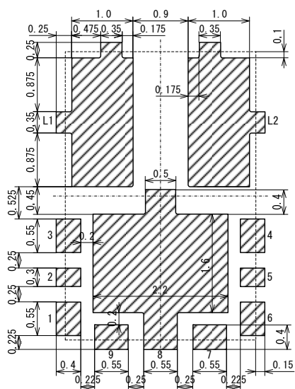
●参考パターンレイアウト/ Reference Pattern Layout
